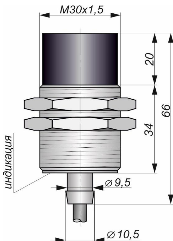
Габаритный чертеж
